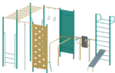
Спортивный комплекс 0770 5280 x 3790 | 2800 9680 x 8180 7-14 2730
