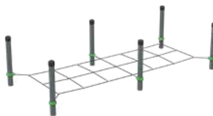
Высокий шаг 1512 4397 x 1973 | 1120 7250 x 4810 7-14 270
