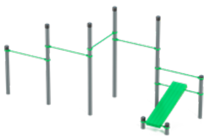
Спортивное оборудование 1720 5250 x 1530 | 2600 8260 x 4960 7+ 1900
