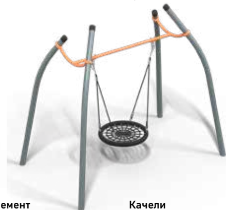
Игровой элемент 0458 2420 x 150 | 1490 4550 x 2200 👤 3-14 🏃 1490
